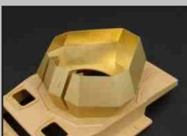
HLX48248 WIRBELWIND turret PE parts for Tamiya kit
